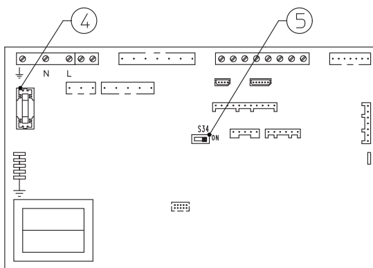
Elektronická doska
