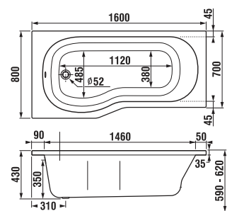
inštalčné rozmery vstavanej vane
